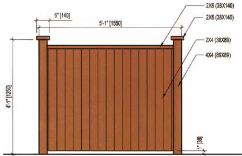
ÉLÉVATION SCHÉMATIQUE – ÉCRAN
