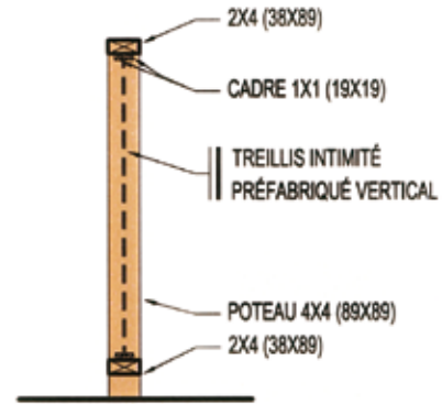
DÉTAIL – POTEAU
