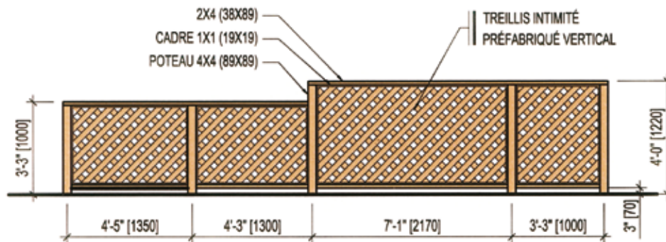
ÉLÉVATION SCHÉMATIQUE – ÉCRAN
