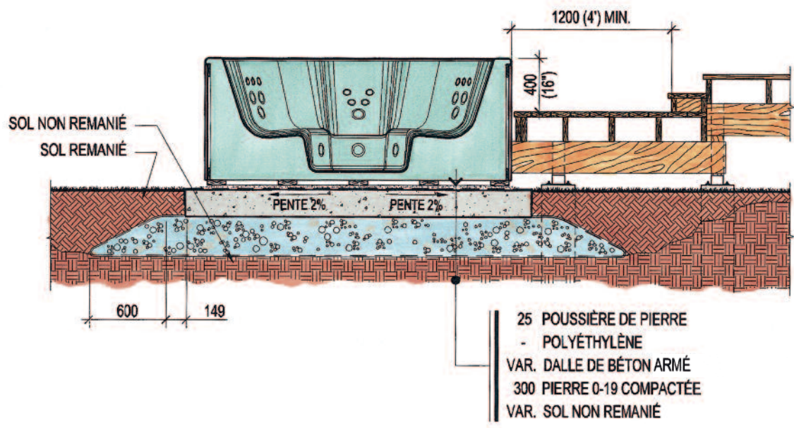
COUPE TYPE - SPA SUR SOCLE DE BÉTON ET TERRASSE EN BOIS
